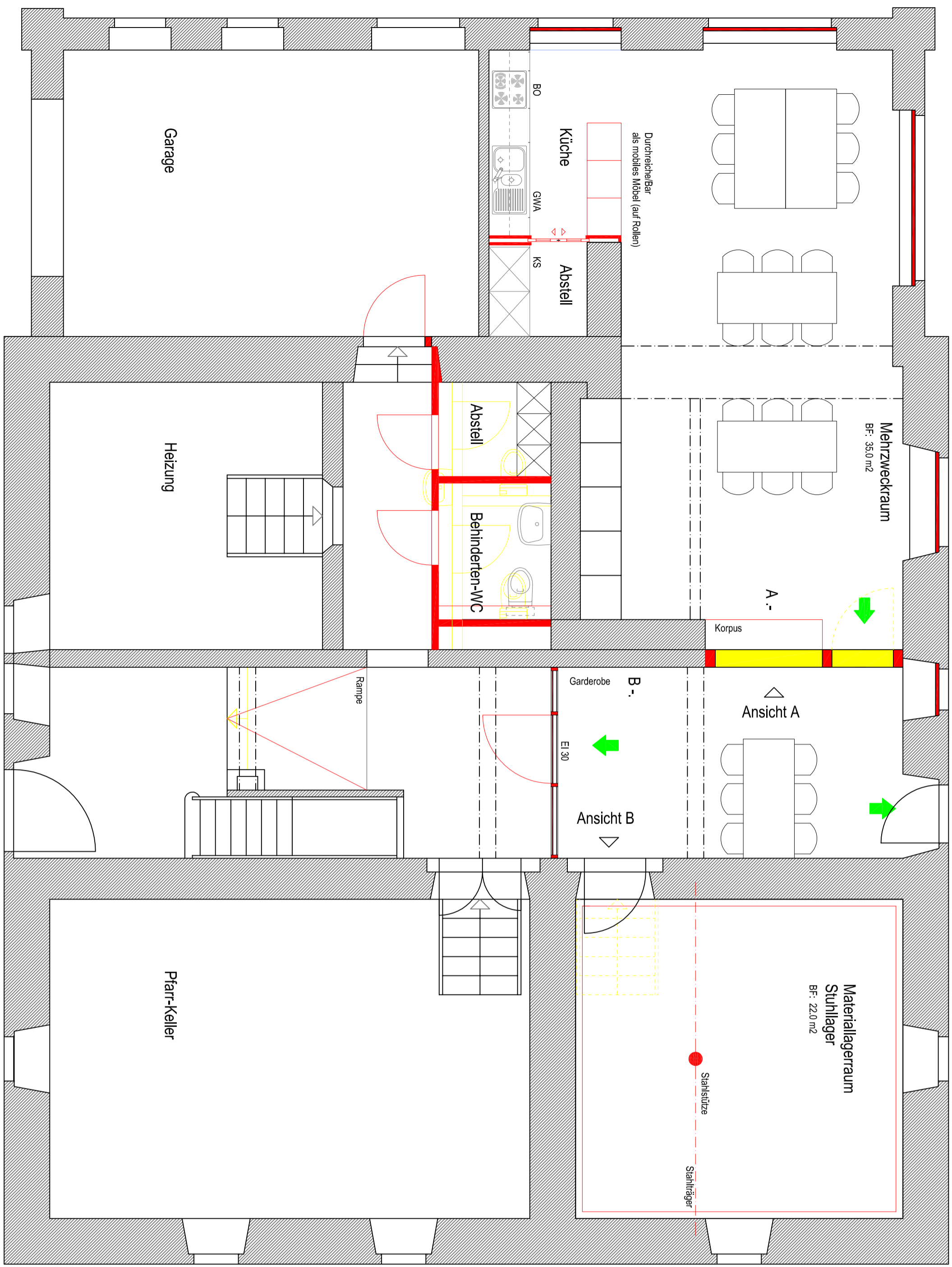
Erdgeschossgrundriss
